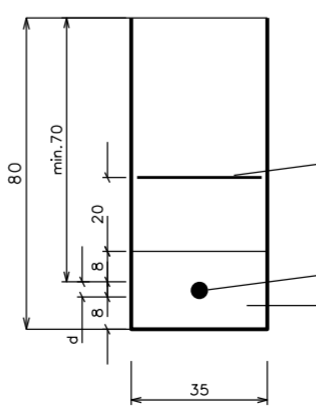
ULOŽENÍ KABELU NN VOLNÝ TERÉN
