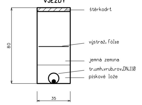
ULOŽENÍ KABELU NN V JEZDY
